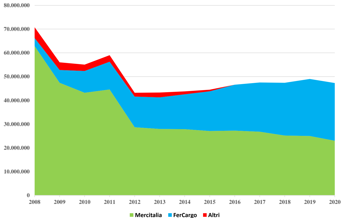
Trasporto ferroviario merci. Andamento Treni/km 2008-2020
